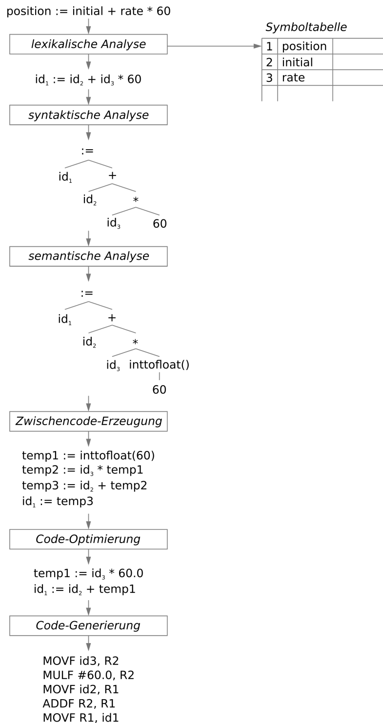
Abbildung 8.2. Schrittweise Übersetzung einer Zuweisung.
