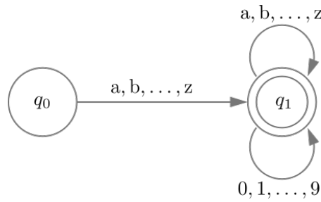
Abbildung 8.3. Deterministischer endlicher Automat, der eine Menge zulässiger Variablenamen erkennt.
