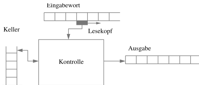
Abbildung 8.5. Schematische Darstellung der Funktionsweise eines Kellerautomaten.
