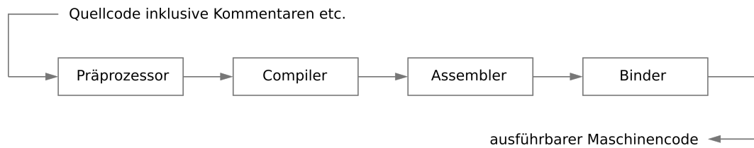
Abbildung 8.1. Schritte der Übersetzung eines Programms.
