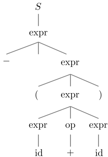
Abbildung 8.4. Strukturbaum zur Formel -(id + id) .
